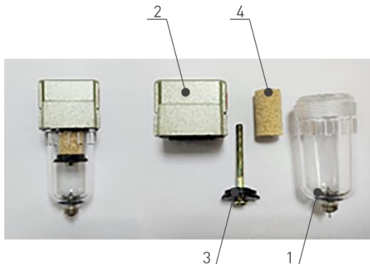
Рисунок 6 – Внешний вид и устройство фильтров.
